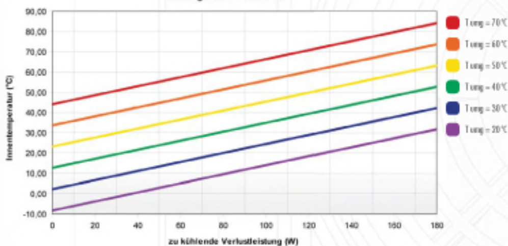
Leistungskennlinie FR-208
