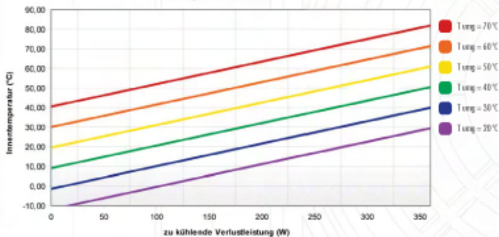
Leistungskennlinie FR-316
