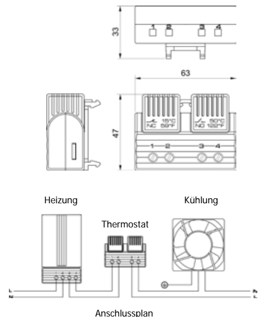
Anschlussplan
