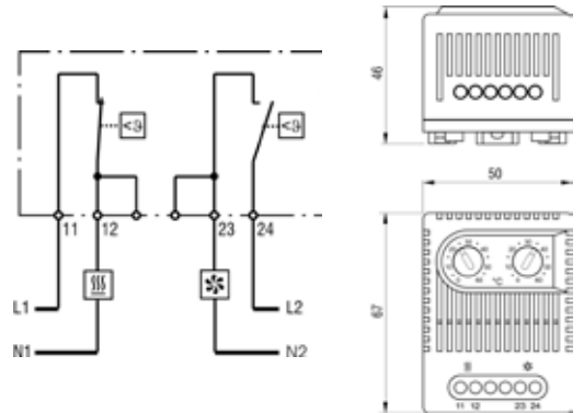
Anschlussplan
