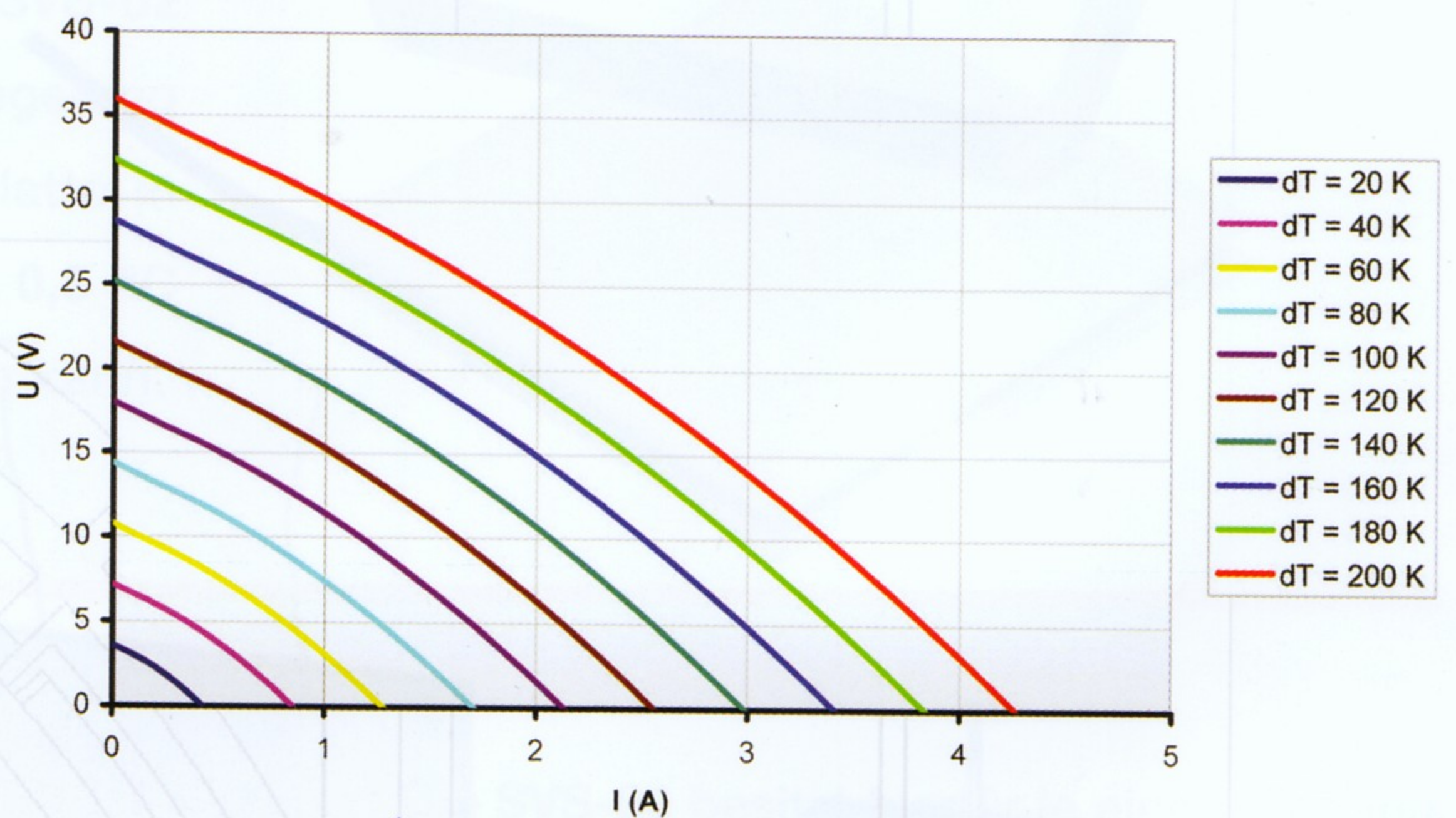
Leistungs-Diagramm Thermogenerator TG-100
