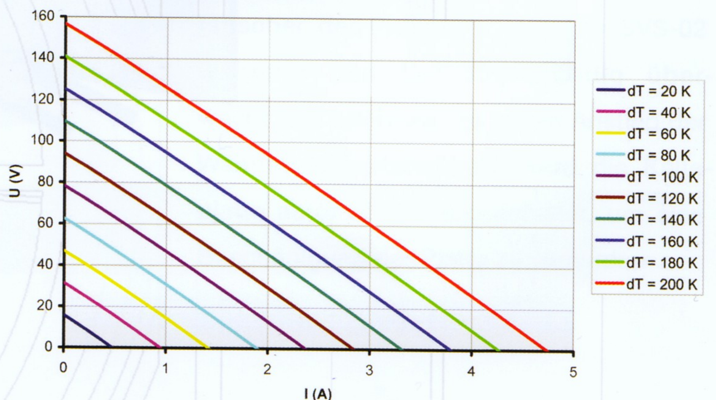
Leistungs-Diagramm Thermogenerator TG-200
